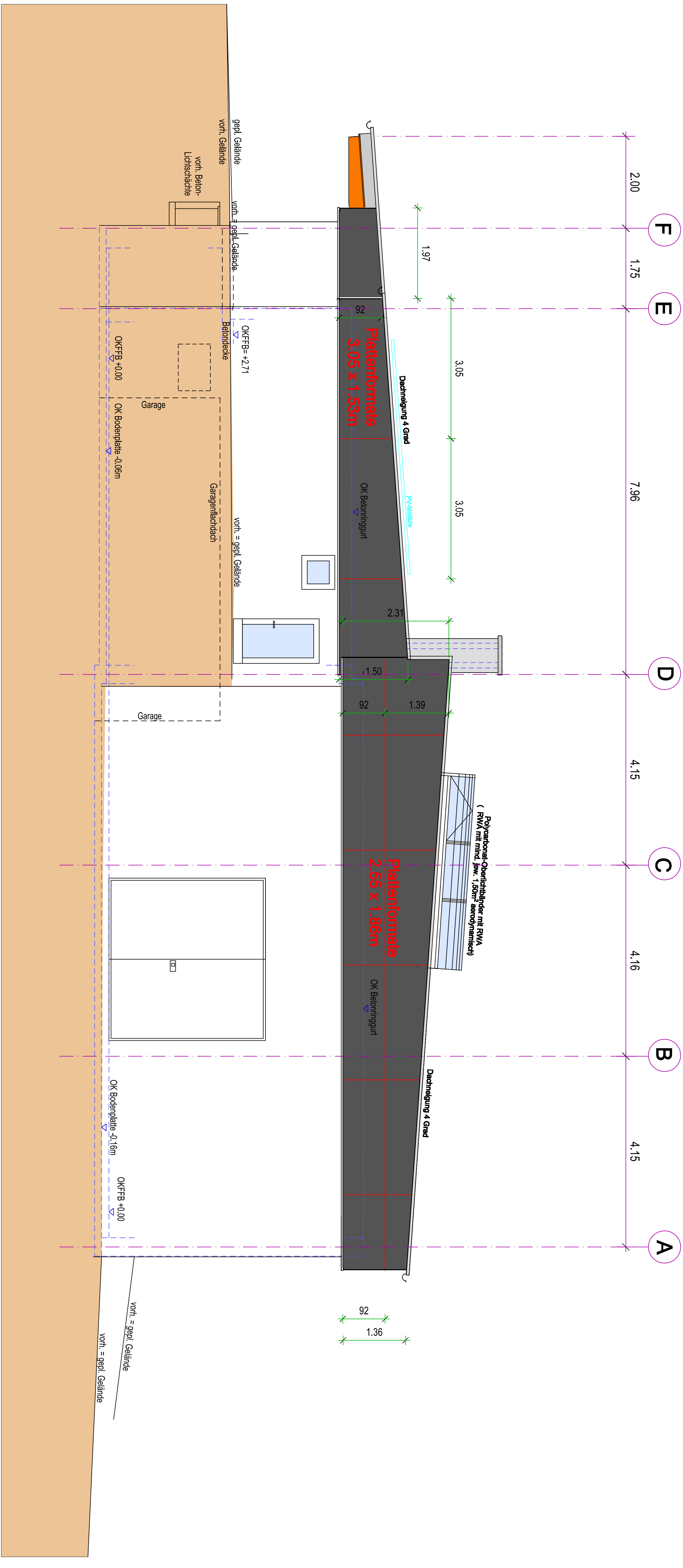
Ansicht Süd M 1:50
